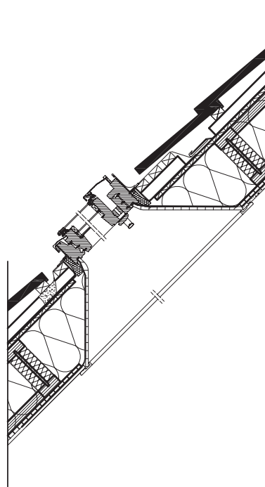
Ortsgang und Gaubenanschluss
