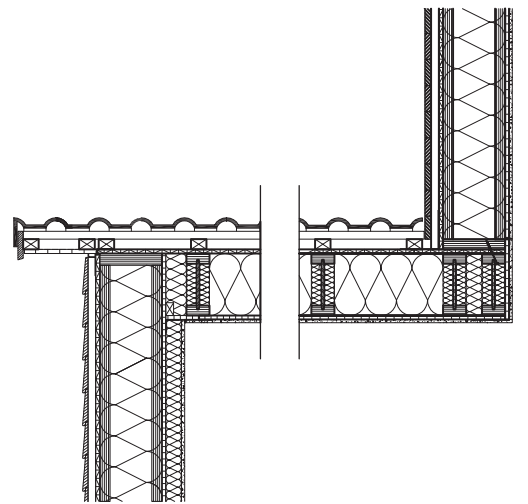
Ortsgang und Gaubenanschluss
